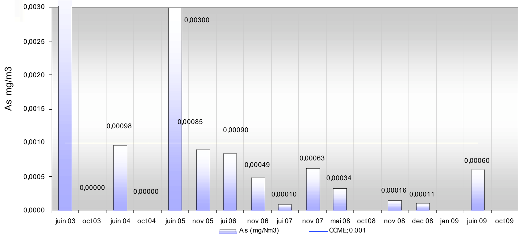
Émissions aux cheminées de l'incinérateur Moyenne des concentrations mesurées pour les émissions d'Arsenic
